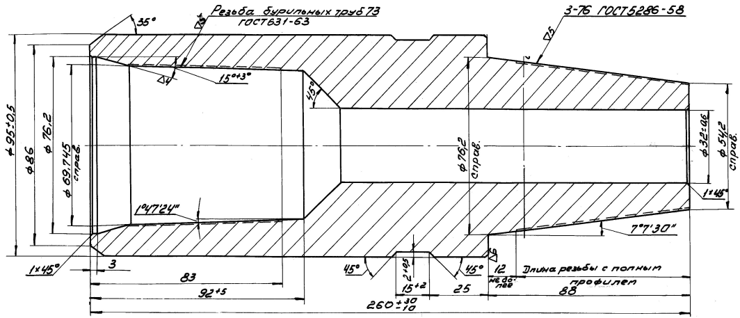
БА15-74.2 - Ниппель
